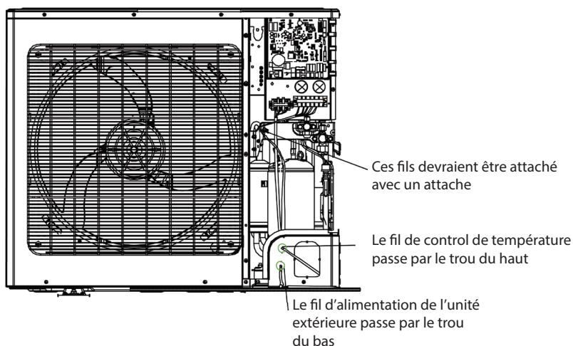
Unité simple phase : GUD36W/A-D(U)
