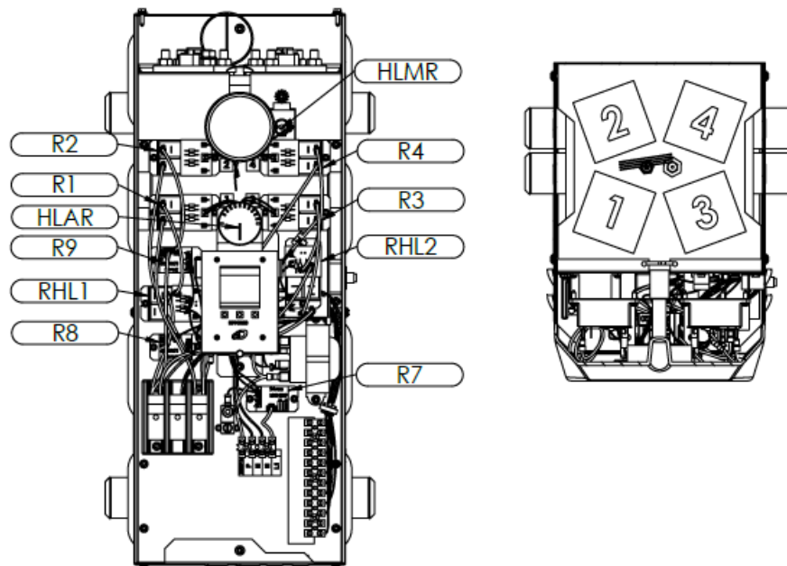
Figure 10: Panneau électrique
