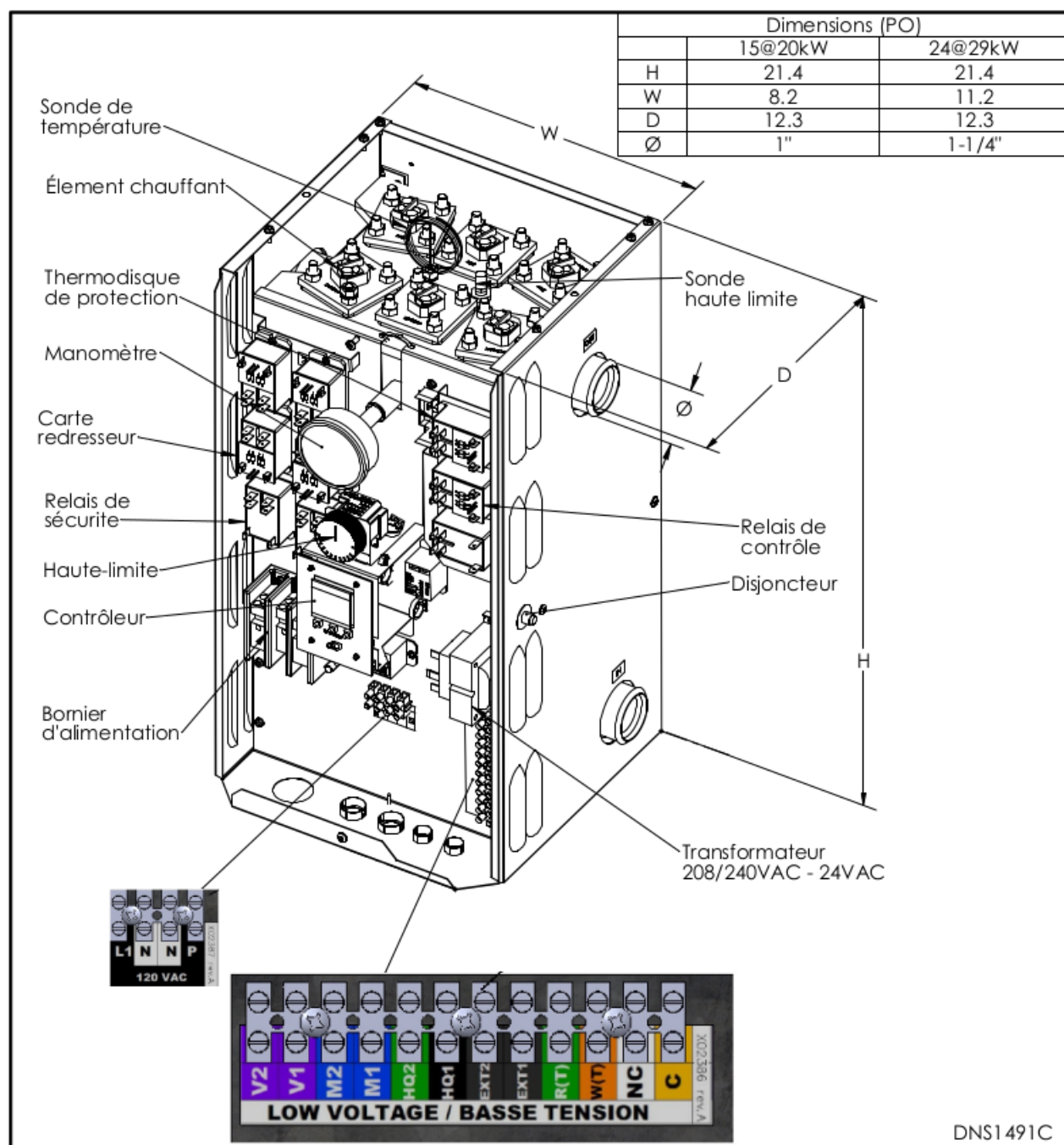
Figure 4: Composantes et dimensions de la chaudière
