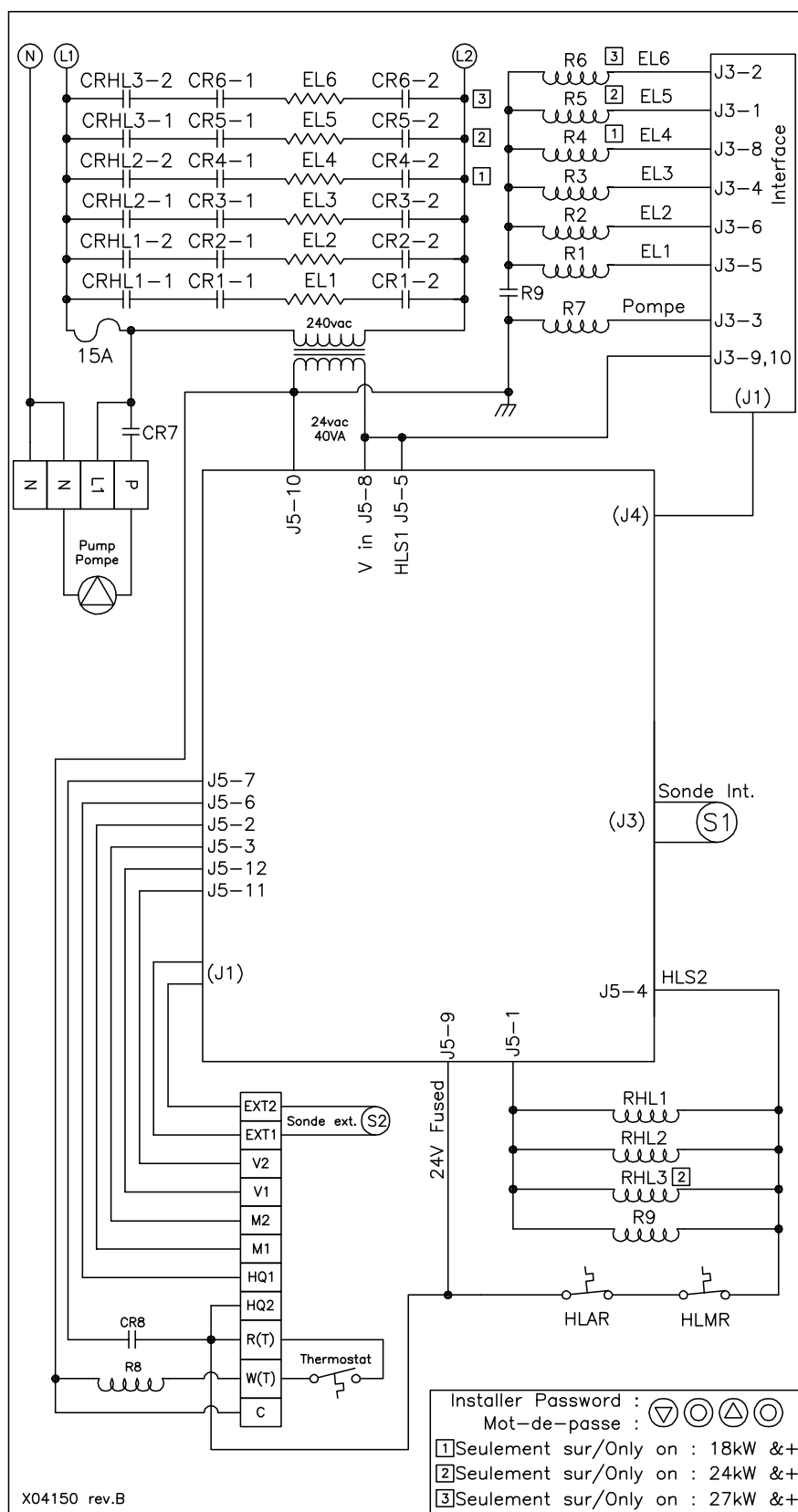
Figure 9: Diagramme électrique
