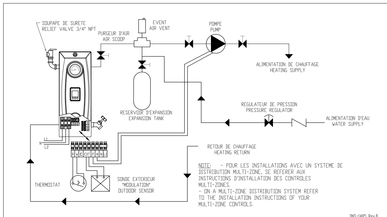
Figure 5: Schéma type d'une installation à une zone
