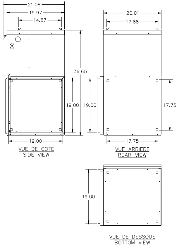
Figure 9 : Dimensions de la fournaise
