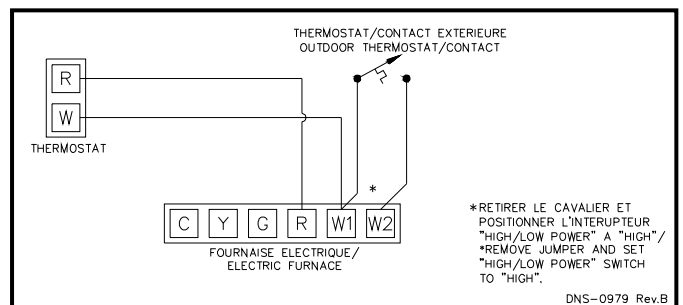
Figure 6 : Thermostat 1-stage avec contrôle extérieur pour fonctionnement en mode 2-stages, chauffage électrique seulement
