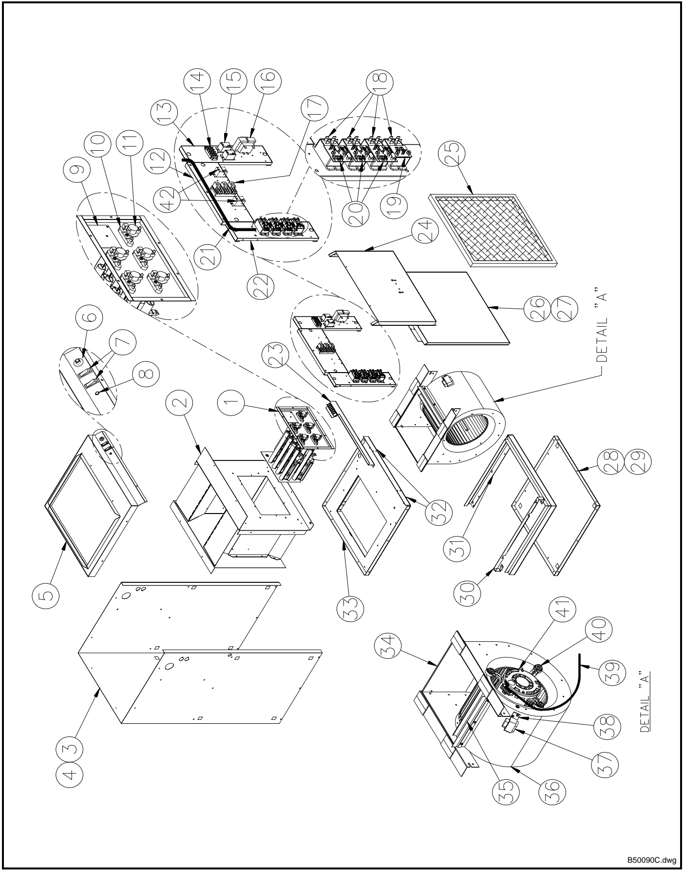
Figure 12 : LISTE DE PIÈCES, Suprême avec moteur 1/3 HP ou 1.0 HP : FEMxx-M2401AM-B ou FEMxx-M2401BM-B
