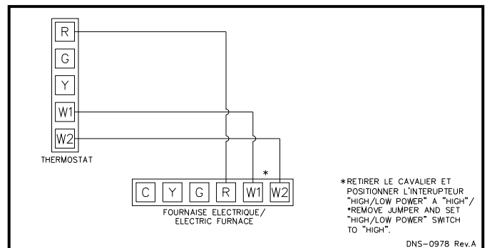
Figure 5 : Thermostat 2-stages, chauffage électrique seulement
