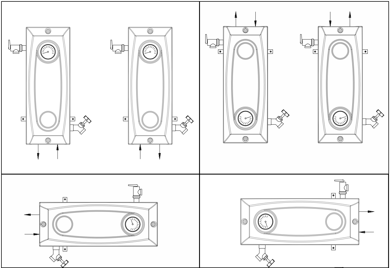
Figure 1 : Configurations de montage
