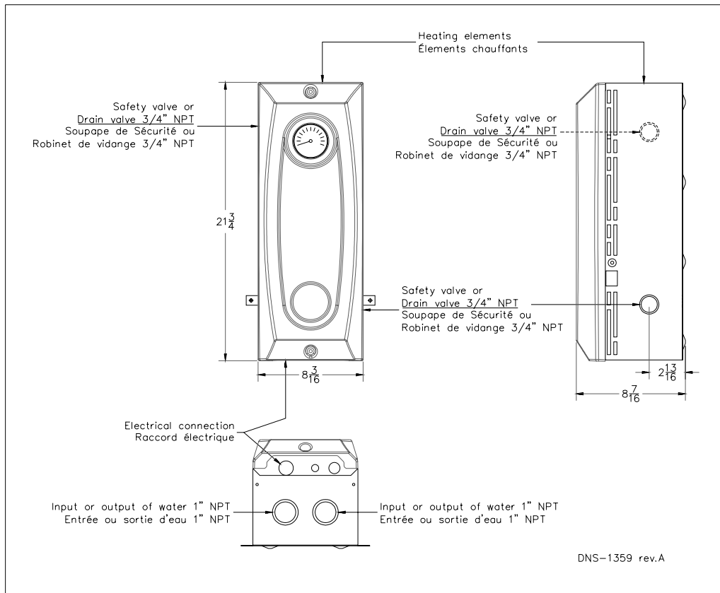
Figure 3 : Dimensions de la chaudière
