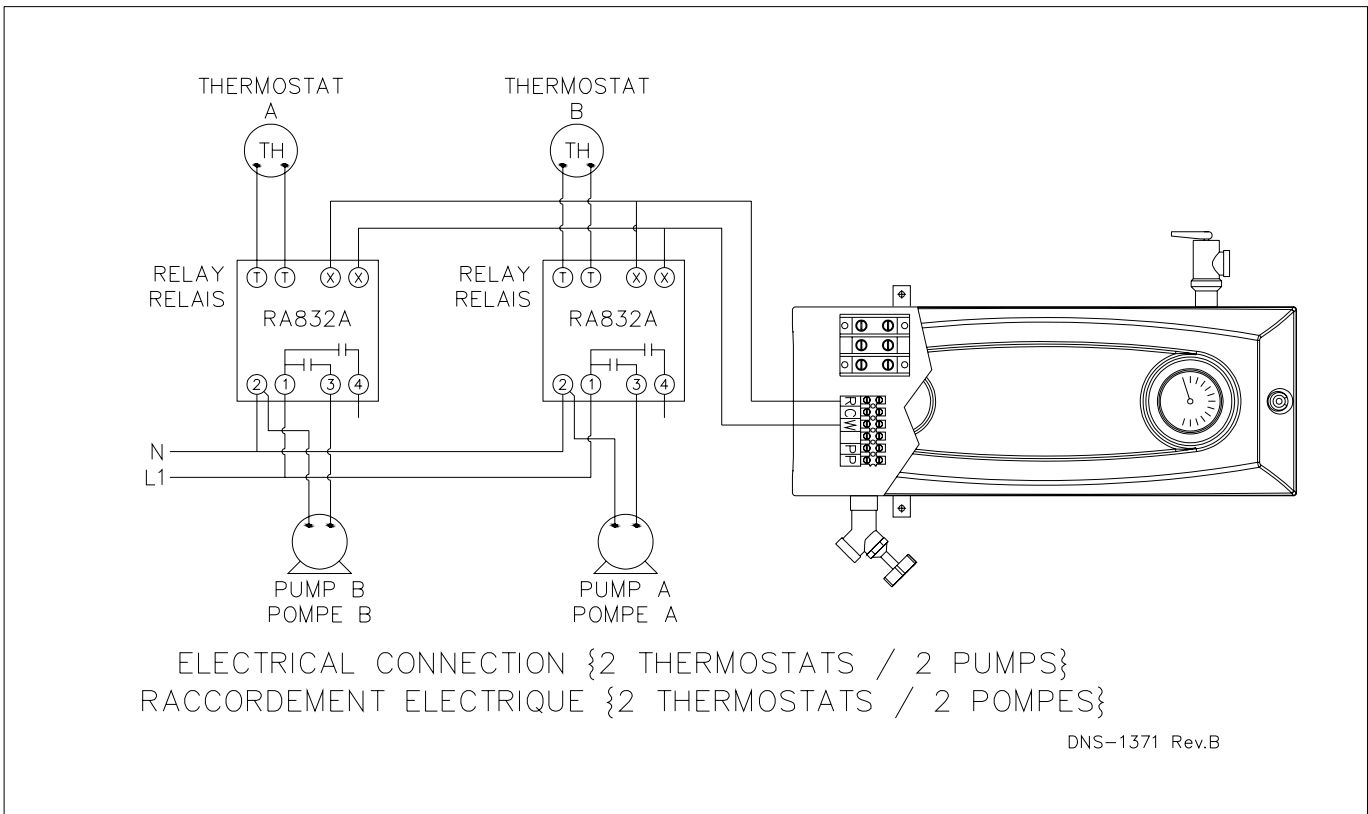
Figure 5 : Diagramme multizone avec plus d'un circulateur
