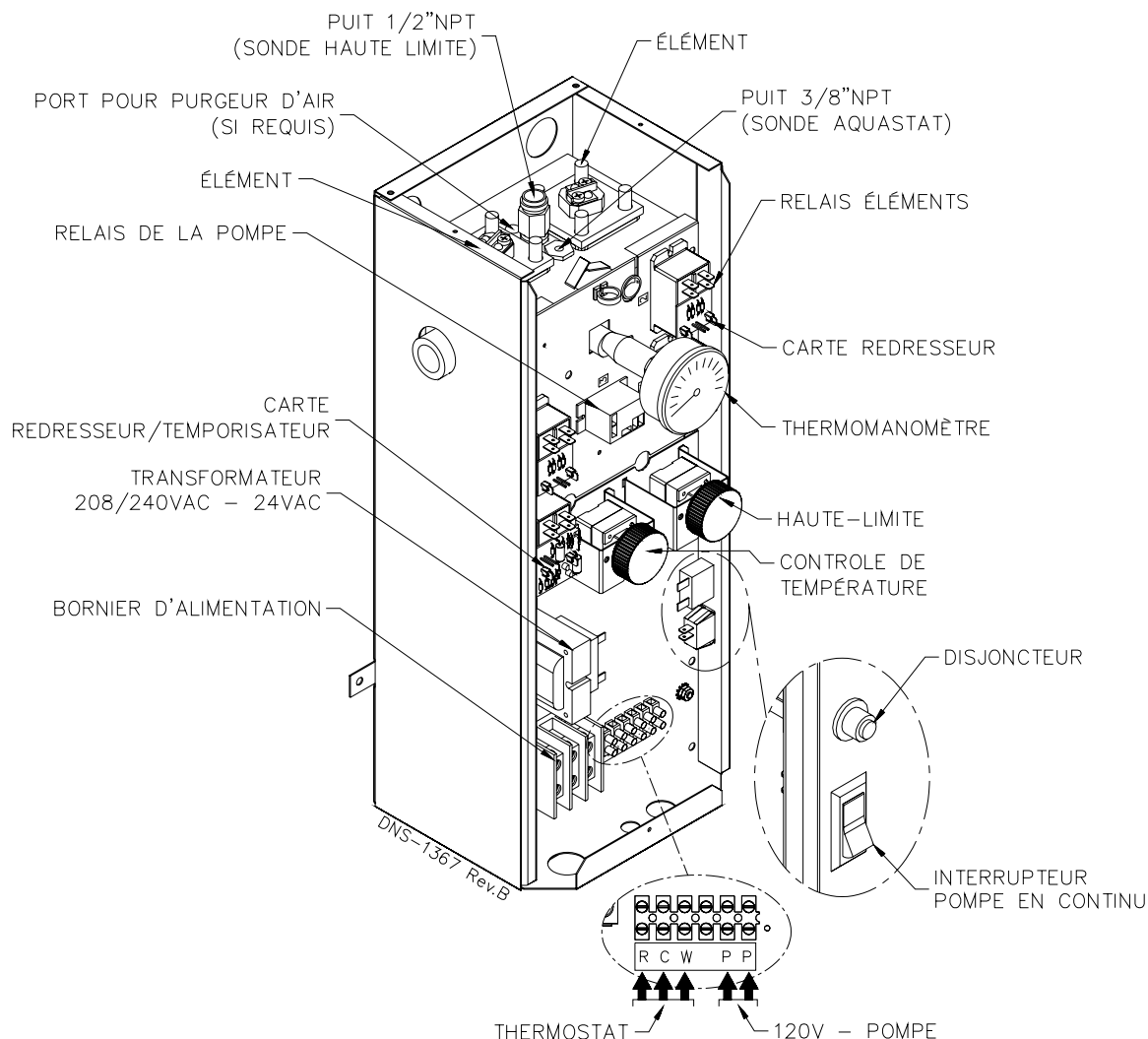
Figure 2 : Composantes de la chaudière
