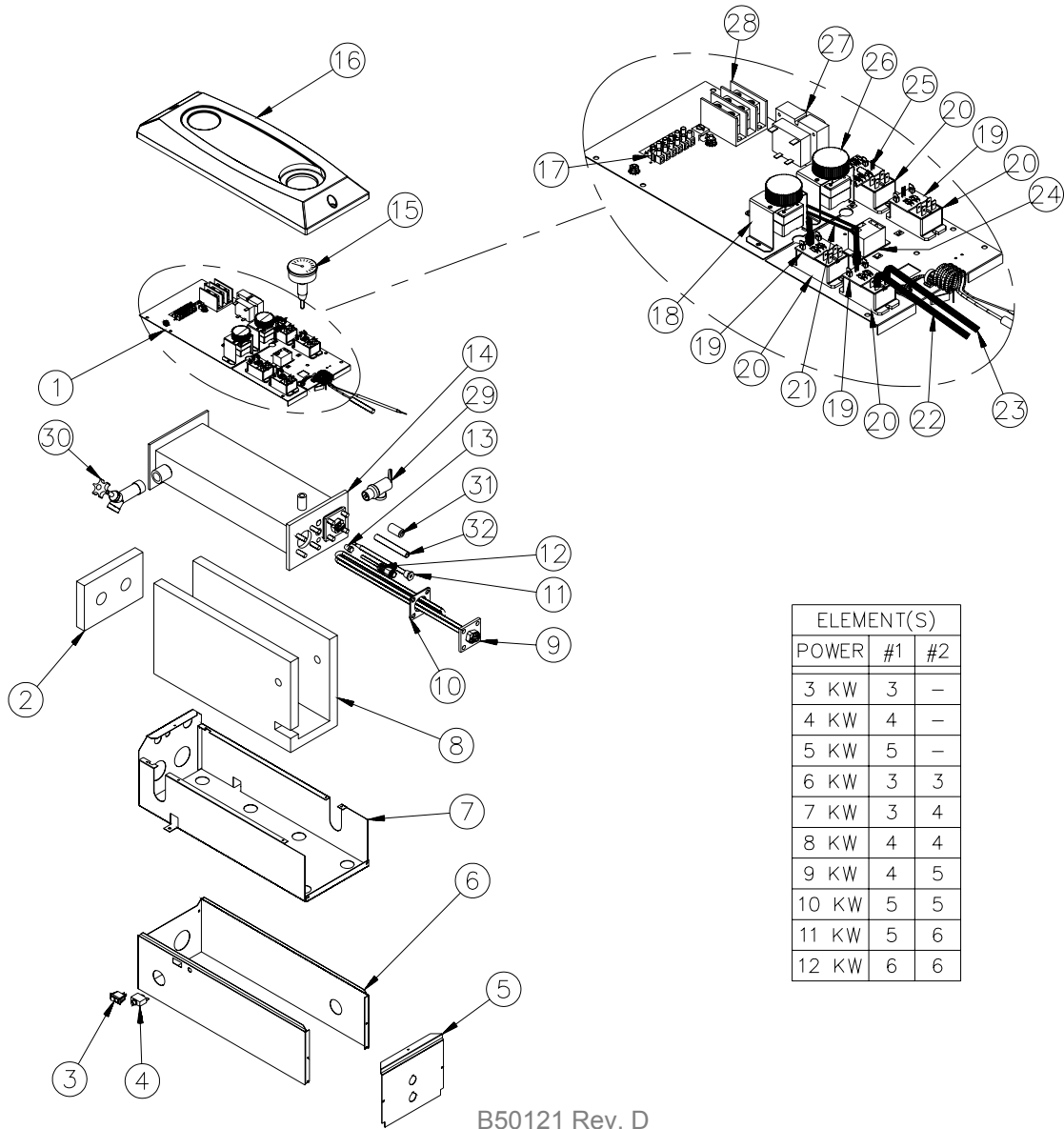
Figure 8 : Vue explosée
