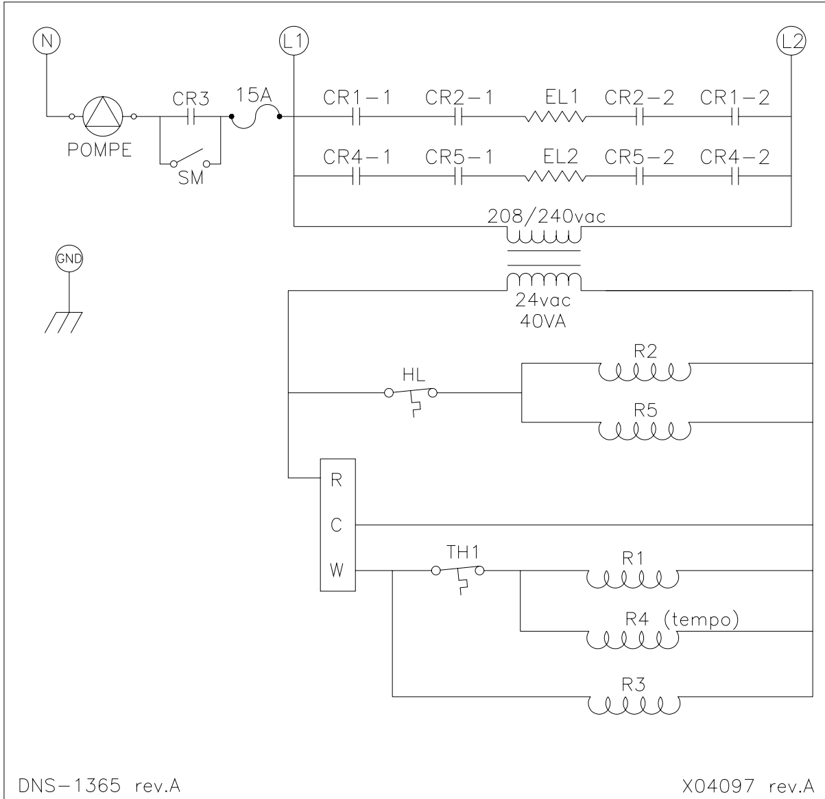
Figure 7 : Diagramme électrique
